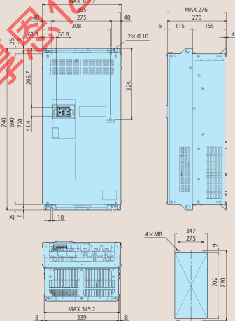
FRN0203E2S-4C
