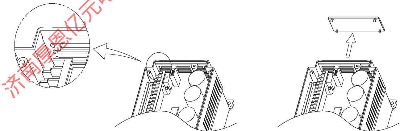
图 2-2-4 通风盖取去方法
