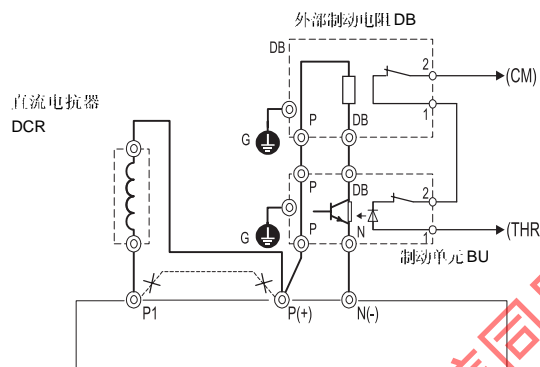
图 2-3-5 连接图
