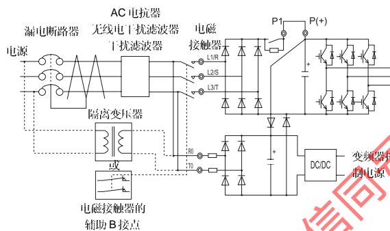
图 2-3-2 控制电源辅助输入的连接方法
