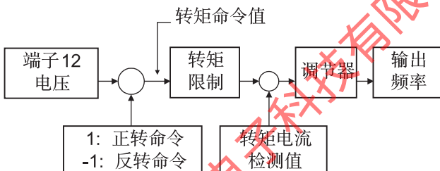
转矩控制框图
