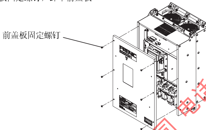
图 1-3-2 卸下前盖板 ( \geq 30\text{kW} )
