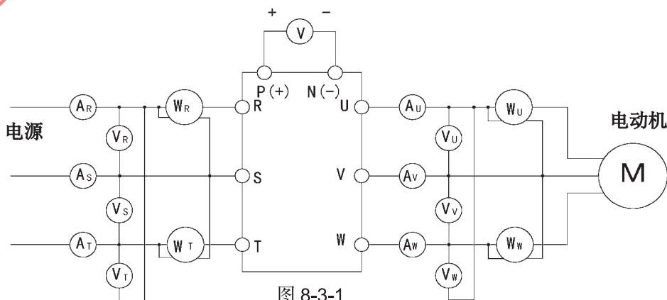
图 8-3-1 表计连接图 8-3
